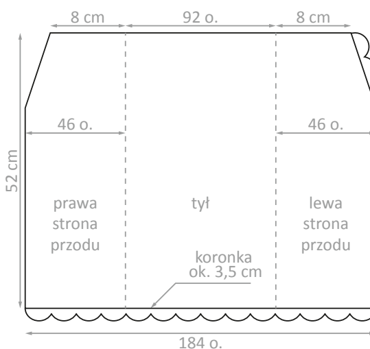
Rys. 1 – Tułów swetra
