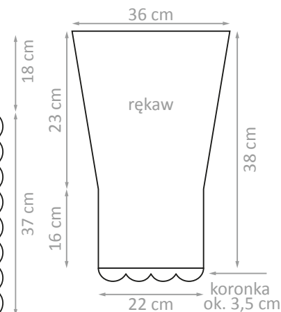
Rys. 2 – Rękaw
