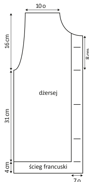
Rys. 2 – Przód
