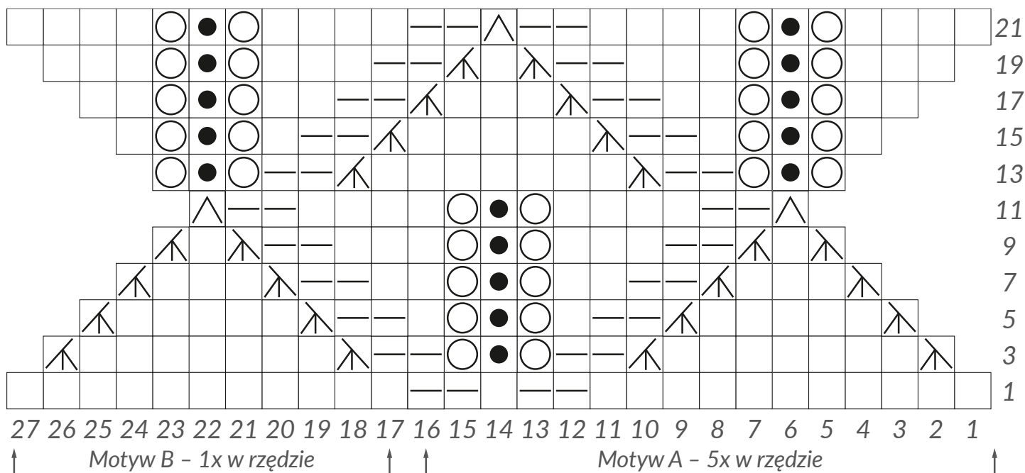
Schemat – Motyw główny serwety
